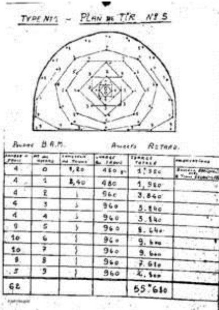
Plan für Bohrarbeiten
